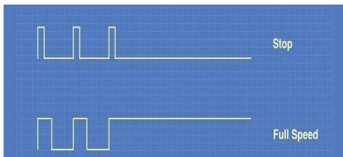
FIG-b): PWM GRAPH
